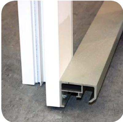
Forklift ramp Passage de chariot Staplerdurchfahrt
